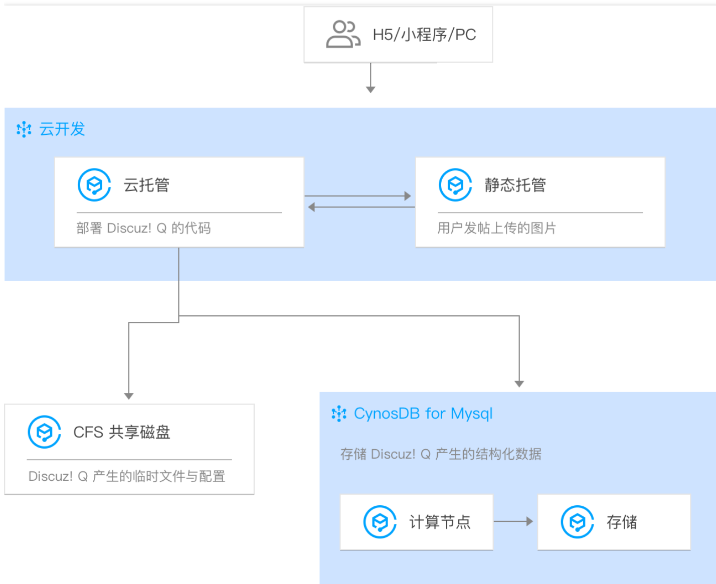
安装 Discuz! Q 资源配置架构图
