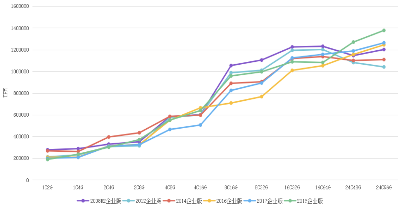
TencentDB for SQL Server 单节点（云 SSD）各版本性能比较
