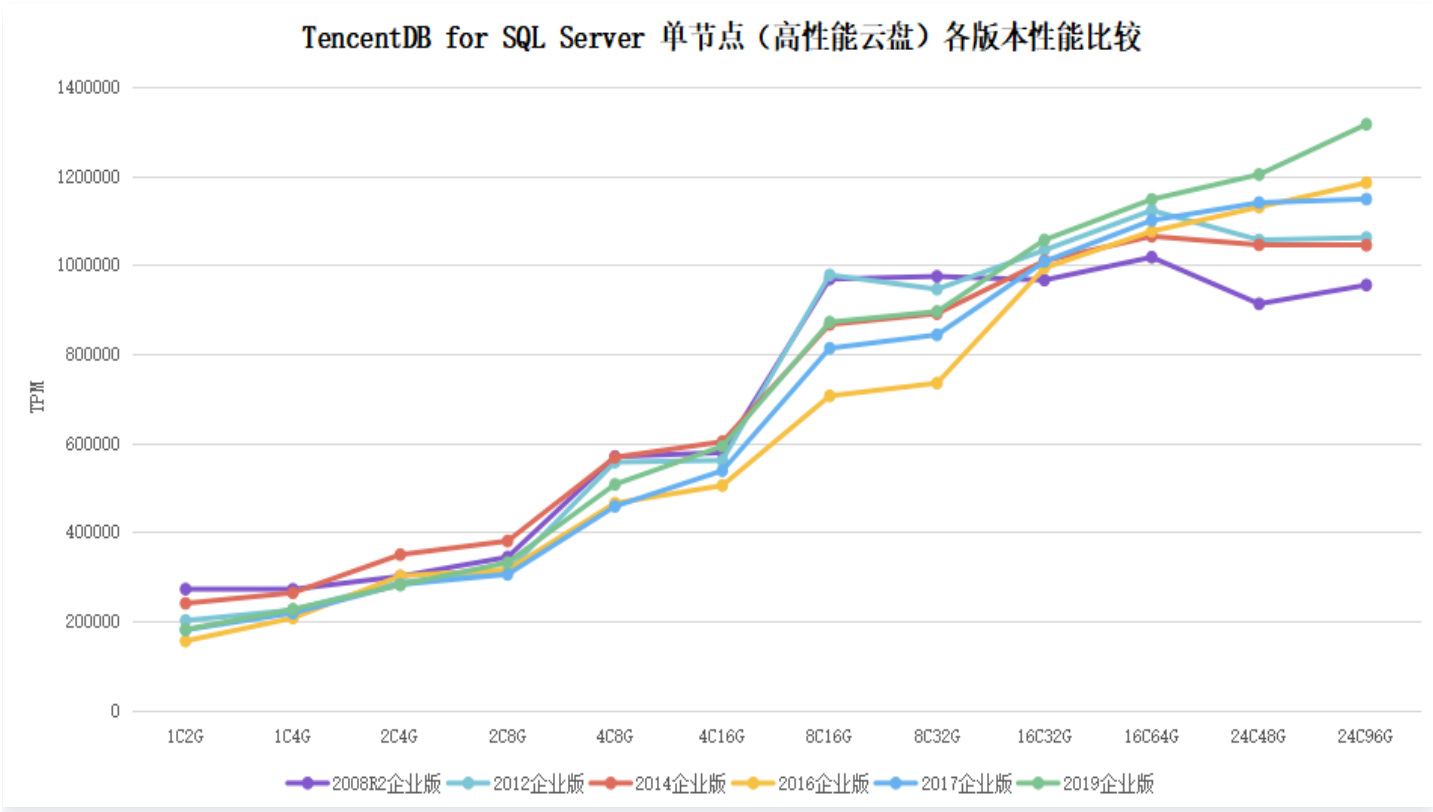
单节点（原基础版-高性能云盘）各版本 TPM 性能对比值
