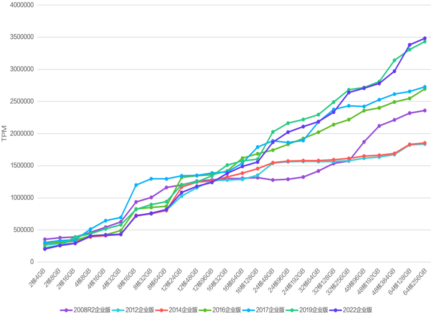
双节点（增强型 SSD 云硬盘）各版本 TPM 性能对比值
