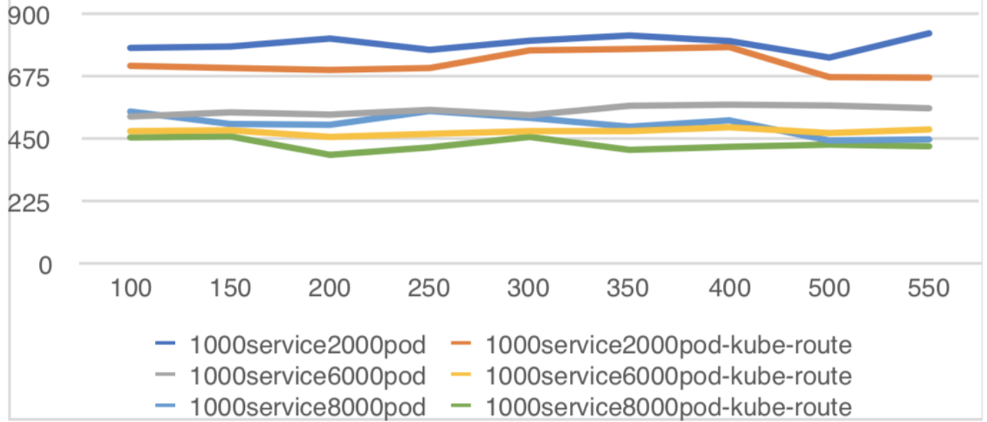
不同pod开启/不开启kube-route时的QPS性能趋势图
